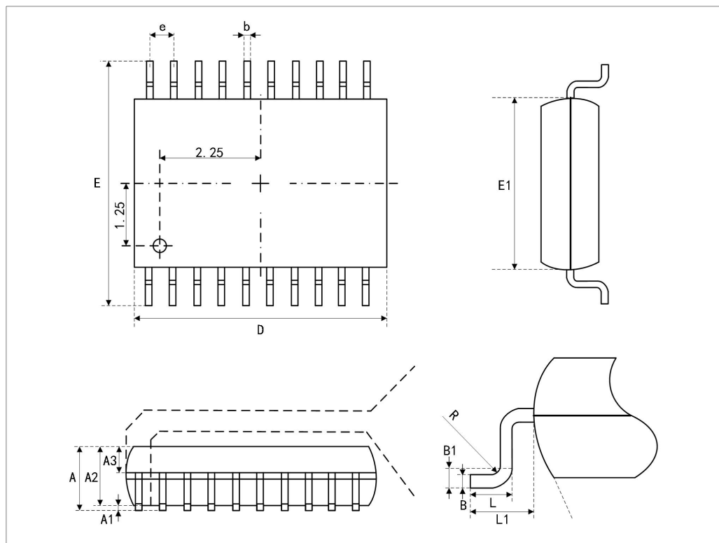
图 6-1 TSSOP20
