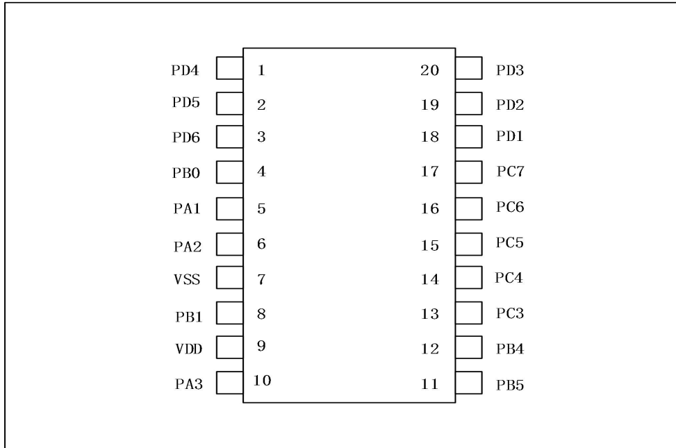
图 3-1 PT32F007x 系列 TSSOP20 封装引脚分布
