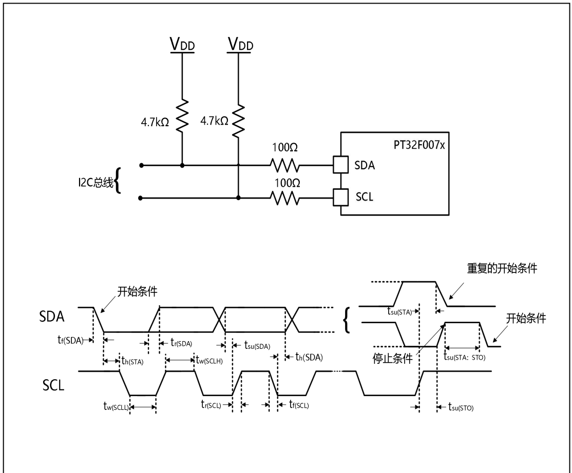
图 5-7 I2C 总线交流波形和测量电路
